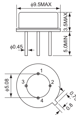
D04 / TO-39
