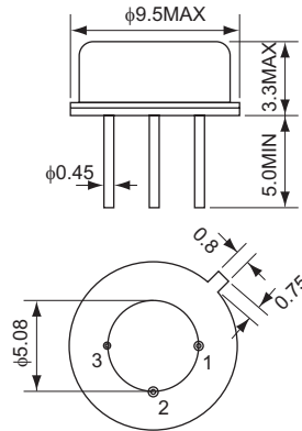
D02 / TO-39
